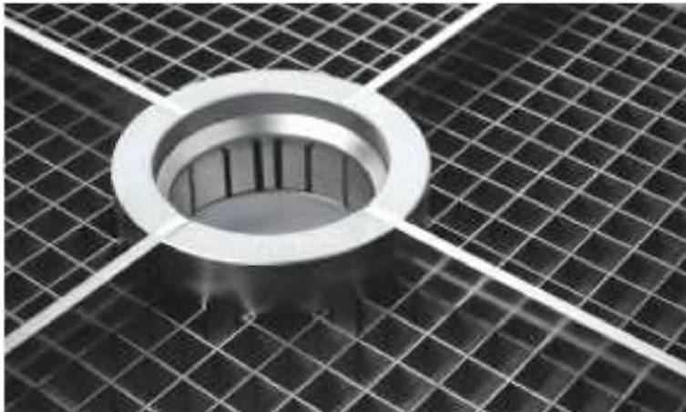
Detailaufnahme Edelstahl Würfelgatter 6 x 6 x 6 mm Detail shot of stainless steel dice screen 6 x 6 x 6 mm
